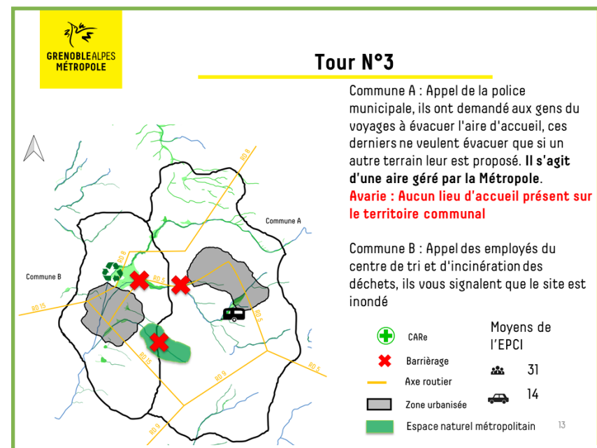
Slika 15: Izvleček scenarija hitrih poplav.
